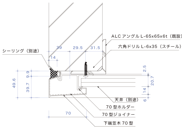
【70用 取付断面図】
