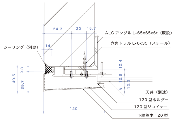
【120用 取付断面図】
